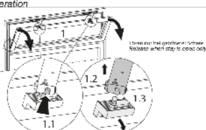
Abb. 15: Flügel sichern/Bedienung Fig. 15: Securing the sash/Operation
