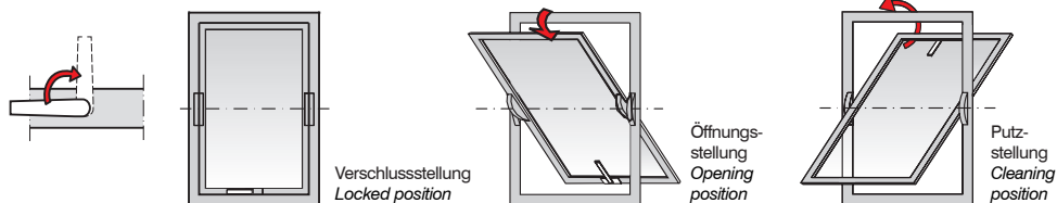
Abb.10: Schwingfenster Fig.10: Horizontal pivot windows
