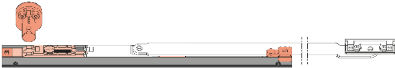
Abb.36: Einstellung Öffnungsbegrenzer abschließbar Fig.36: Positions opening limiter lockable
